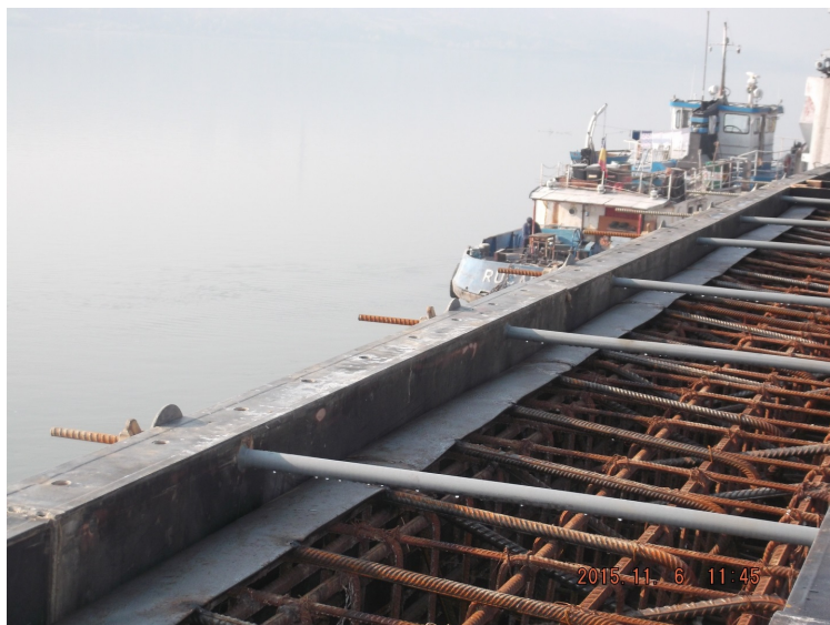
Cofrare grindă de coronament
